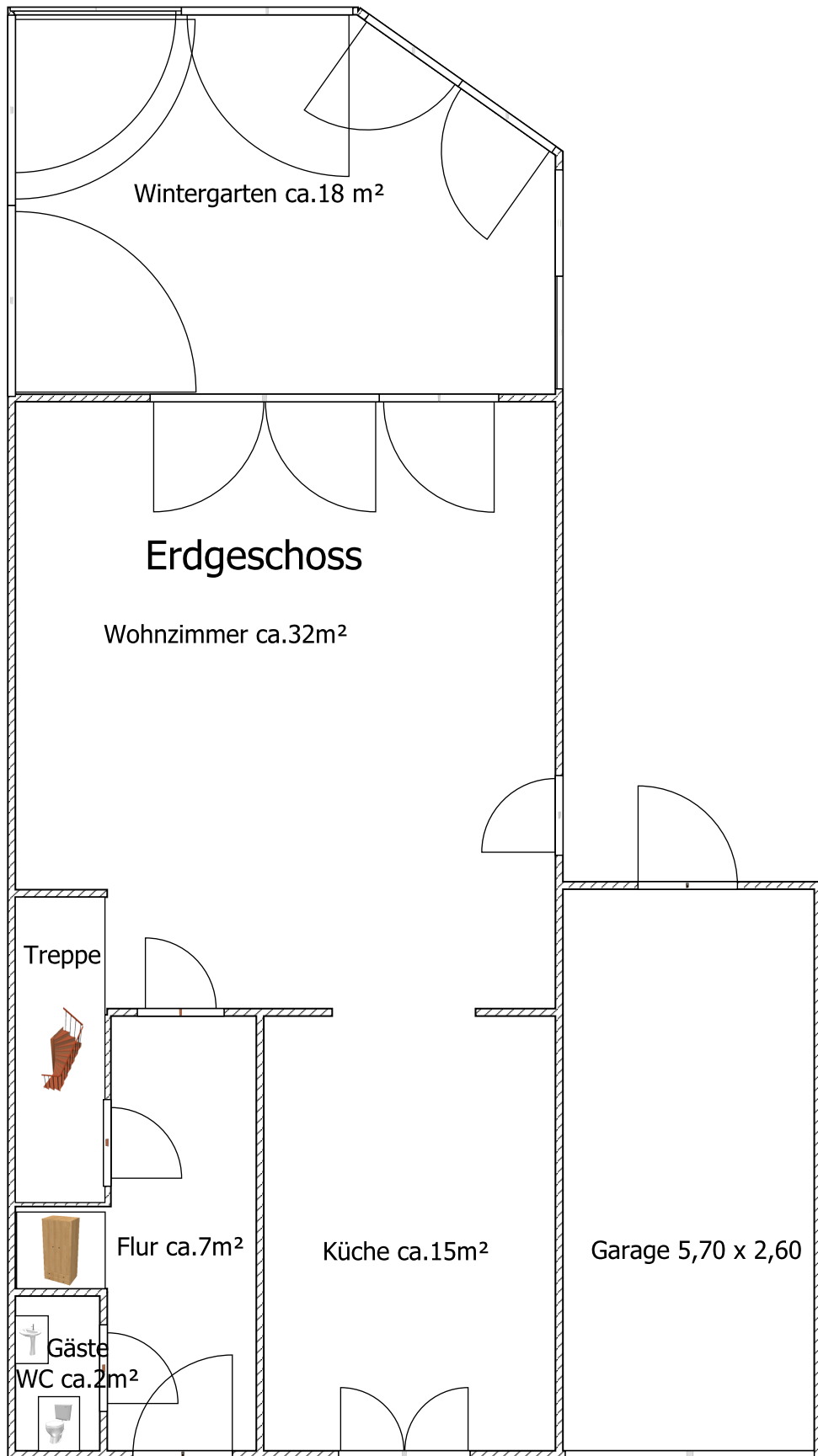
maßstabsähnlicher Grundriss
